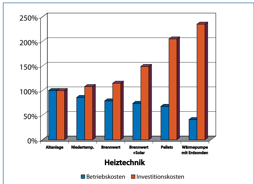
Abb. 2 Investitions- und Betriebskostenvergleich unterschiedlicher Heiztechniken
