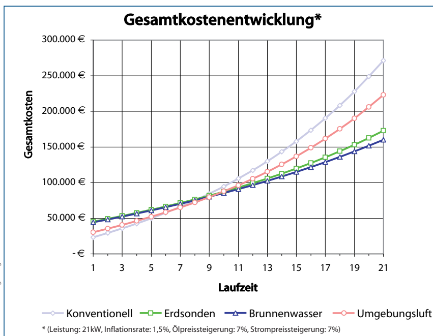
Abb. 3 Gesamtkostenvergleich unterschiedlicher Wärmepumpensysteme unter Berücksichtigung von Preissteigerungen
