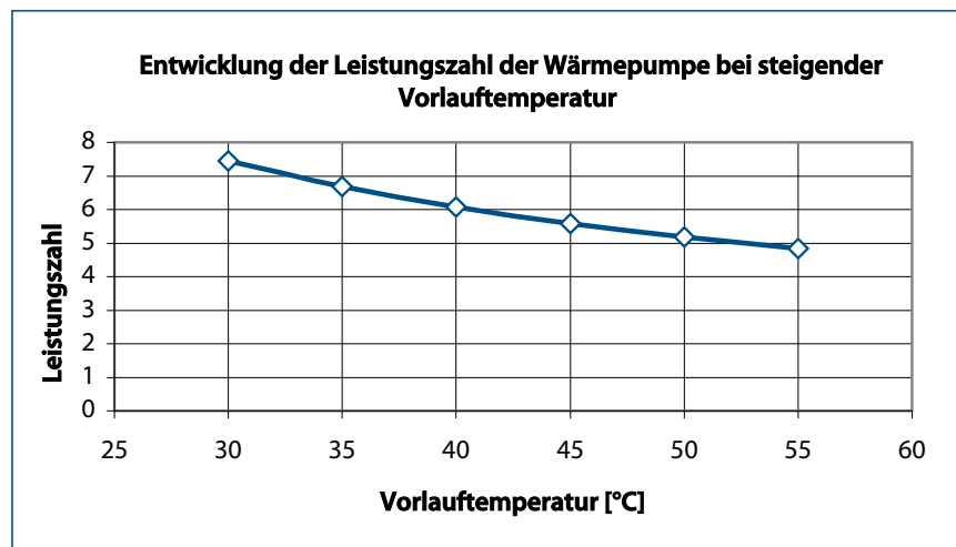
Abb. 4 Effizienz der Wärmepumpenheizung in Abhängigkeit der Vorlauftemperatur
